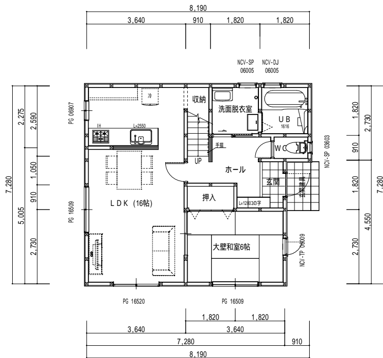
1階平面図 1 / 100
