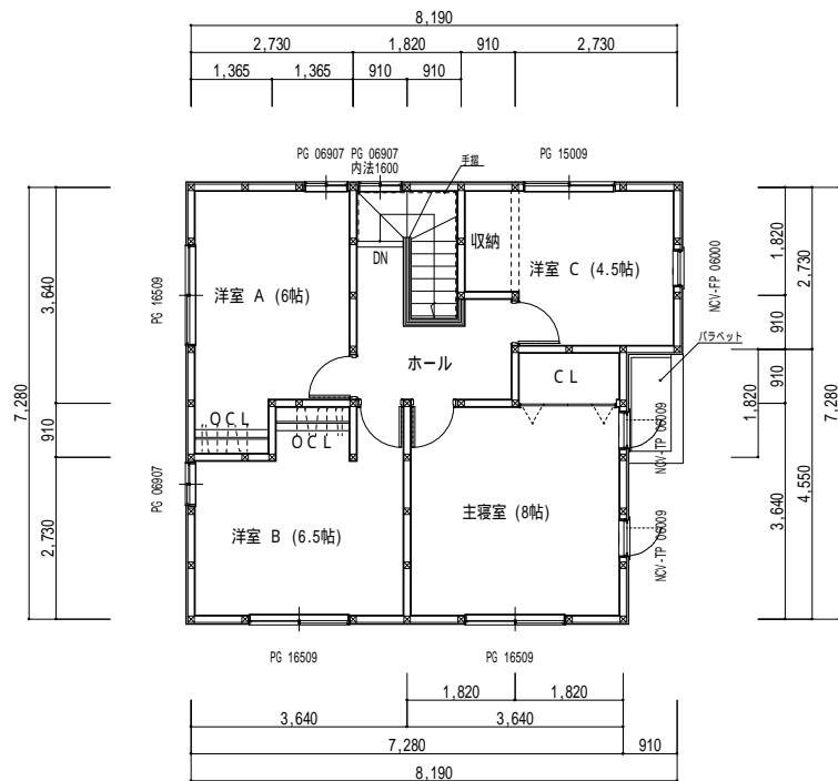
2階平面図 1 / 100
