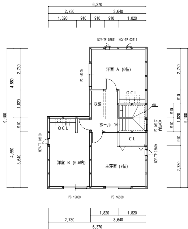
2階平面図 1 / 100
