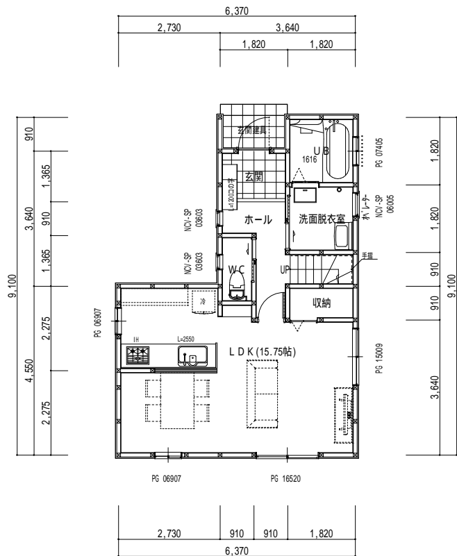
1階平面図 1 / 100
